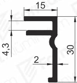
Pr.No: 8597 0,313 kg/m
