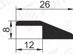
Pr.No: 9483 0,244 kg/m
