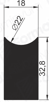
Pr.No:2523 1,465 Kg/m
