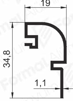
Pr.No: 8813 0,238kg/m
