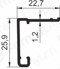
Pr.No: 8862 0,190 kg/m
