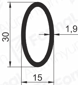
Pr.No: 8707 0,333 kg/m
