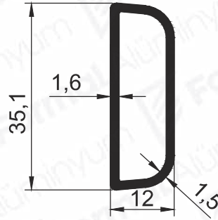
Pr.No: 9545 0,344 kg/m
