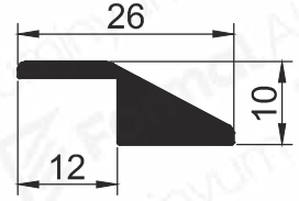
Pr.No: 981 0,280 kg/m
