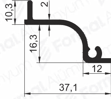
Pr.No: 2248 0,335 kg/m
