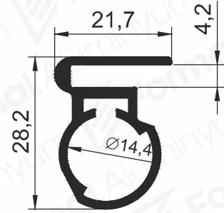
Pr.No: 9584 0,406 kg/m
