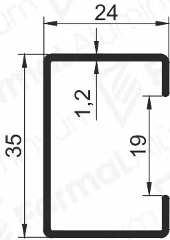
Pr.No:2631 0,300 kg/m
