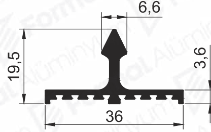
Pr.No: 9820 0,350 kg/m
