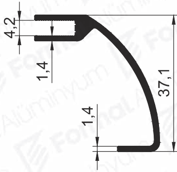
Pr.No: 9583 0,365 kg/m
