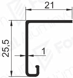
Pr.No: 8580 0,145 kg/m
