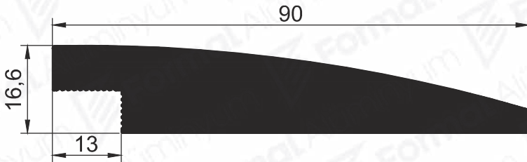
Pr.No: 9901 2,838 kg/m
