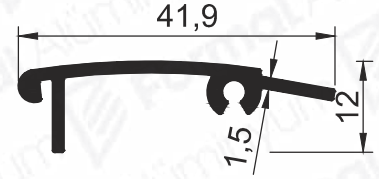
Pr.No: 8625 0,29 kg/m
