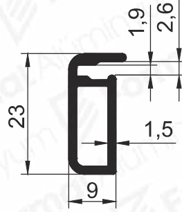
Pr.No: 8511 0,256 kg/m
