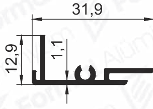
Pr.No: 8814 0,184 kg/m
