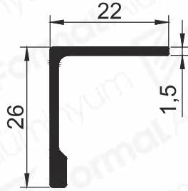
Pr.No: 8650 0,216 kg/m
