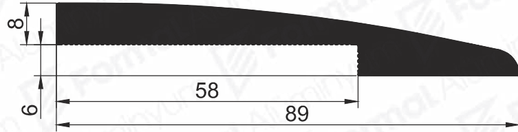
Pr.No:2479 1,665 kg/m
