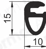
Pr.No: 8742 0,181 kg/m
