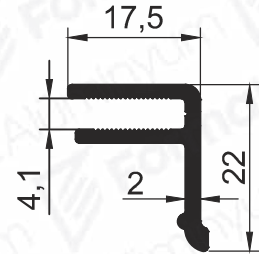
Pr.No: 9367 0,262 kg/m
