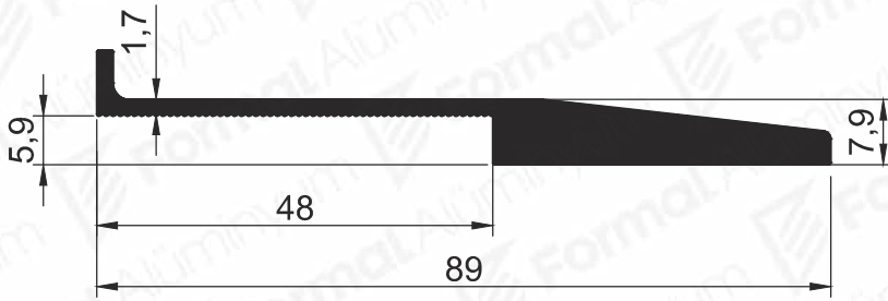
Pr.No: 1946 0,971 kg/m
