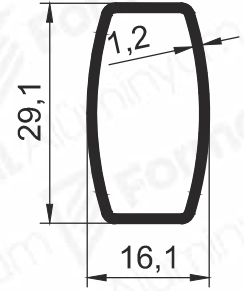
Pr.No: 9267 0,253 kg/m
