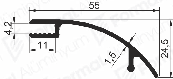
Pr.No: 9418 0,390 kg/m
