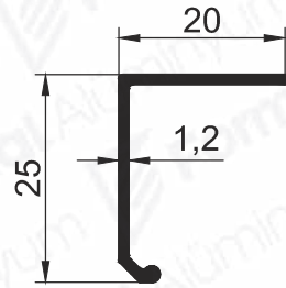
Pr.No: 8905 0,154 kg/m
