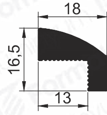
Pr.No: 9904 0,389 kg/m
