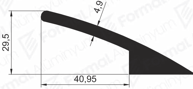
Pr.No:2787 1,306 kg/m
