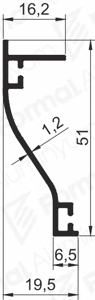
Pr.No:2520 0,294 kg/m
