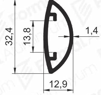
Pr.No: 1236 0,322 kg/m
