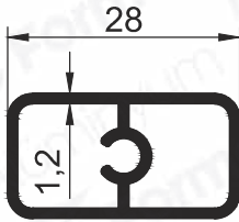
Pr.No: 2235 0,316 kg/m
