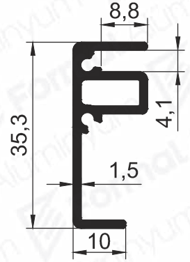
Pr.No:2630 0,34 kg/m
