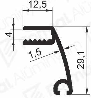
Pr.No: 9382 0,286 kg/m
