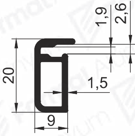
Pr.No: 8096 0,231 kg/m
