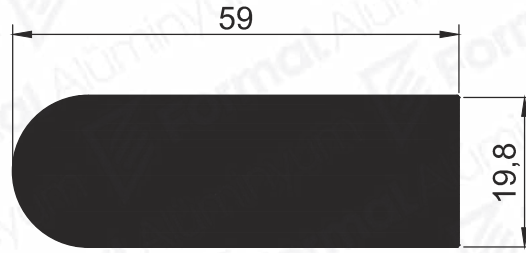
Pr.No: 1984 3,081 kg/m
