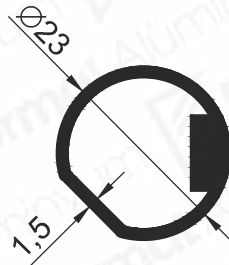
Pr.No: 2454 0,364 kg/m
