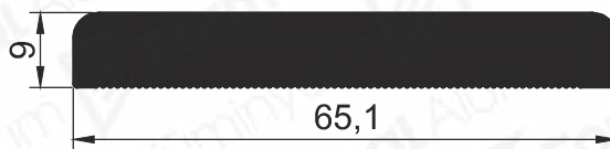
Pr.No:2649 1,55 kg/m
