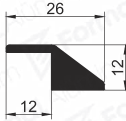
Pr.No: 9819 0,338 kg/m
