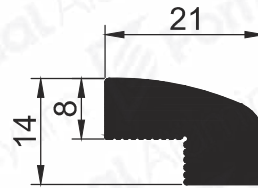
Pr.No: 1969 0,531 kg/m
