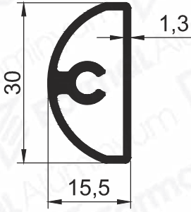
Pr.No: 2455 0,363 kg/m
