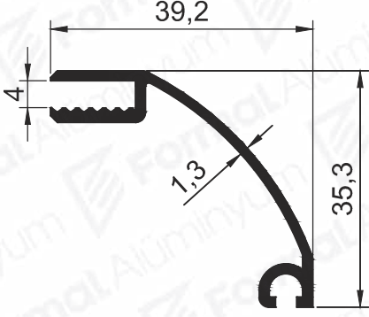
Pr.No: 8137 0,355 kg/m
