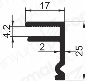
Pr.No: 9240 0,308 kg/m
